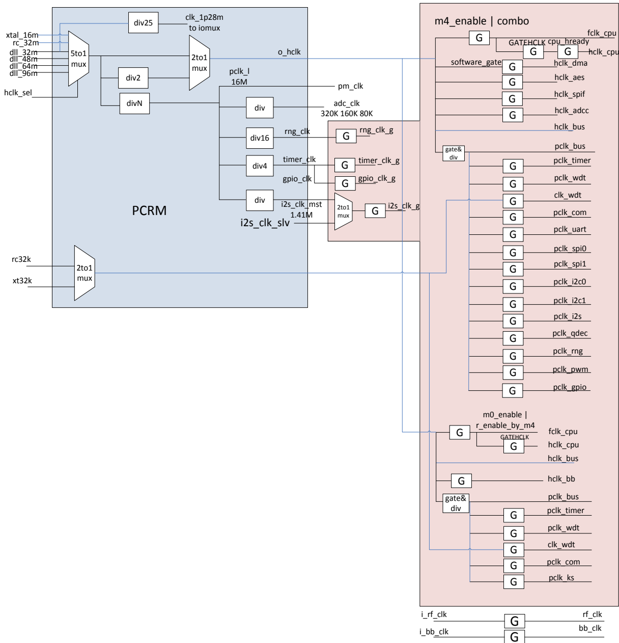
图 9：时钟结构图
