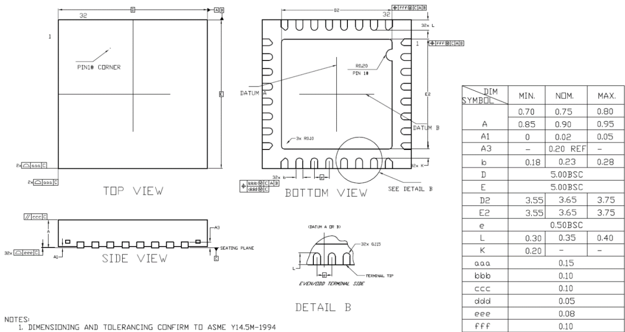
图 15：QFN32 封装尺寸
