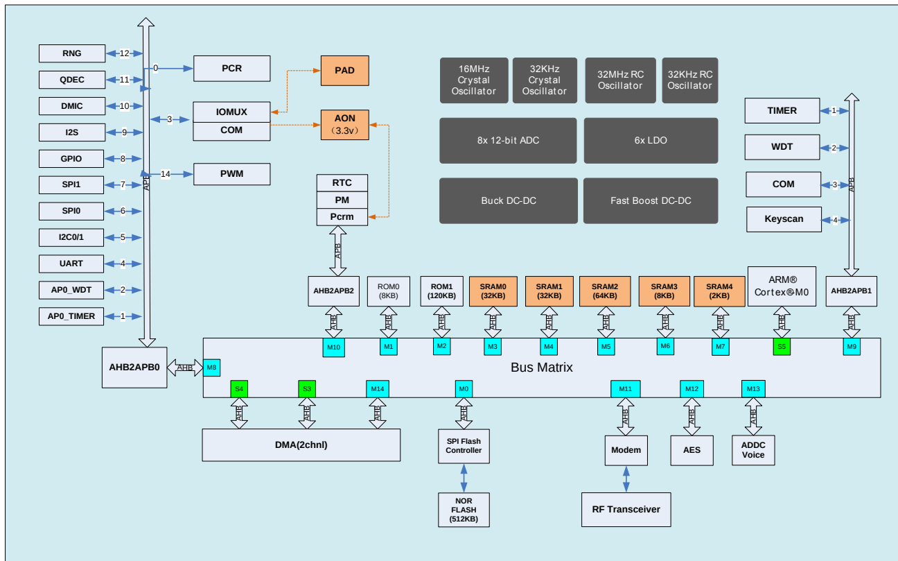
图 1 : CMT4502 框图
