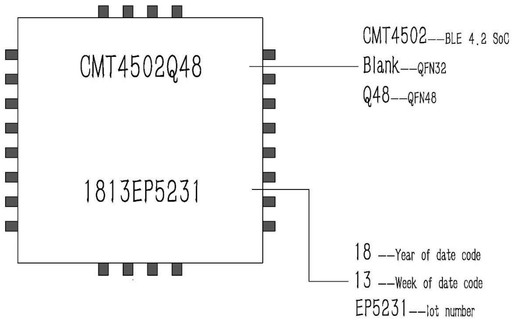
图 14 : 芯片打标
