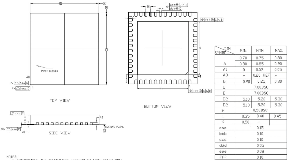
图 16：QFN48 封装尺寸
