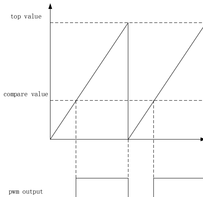
图 11: PWM 图示
